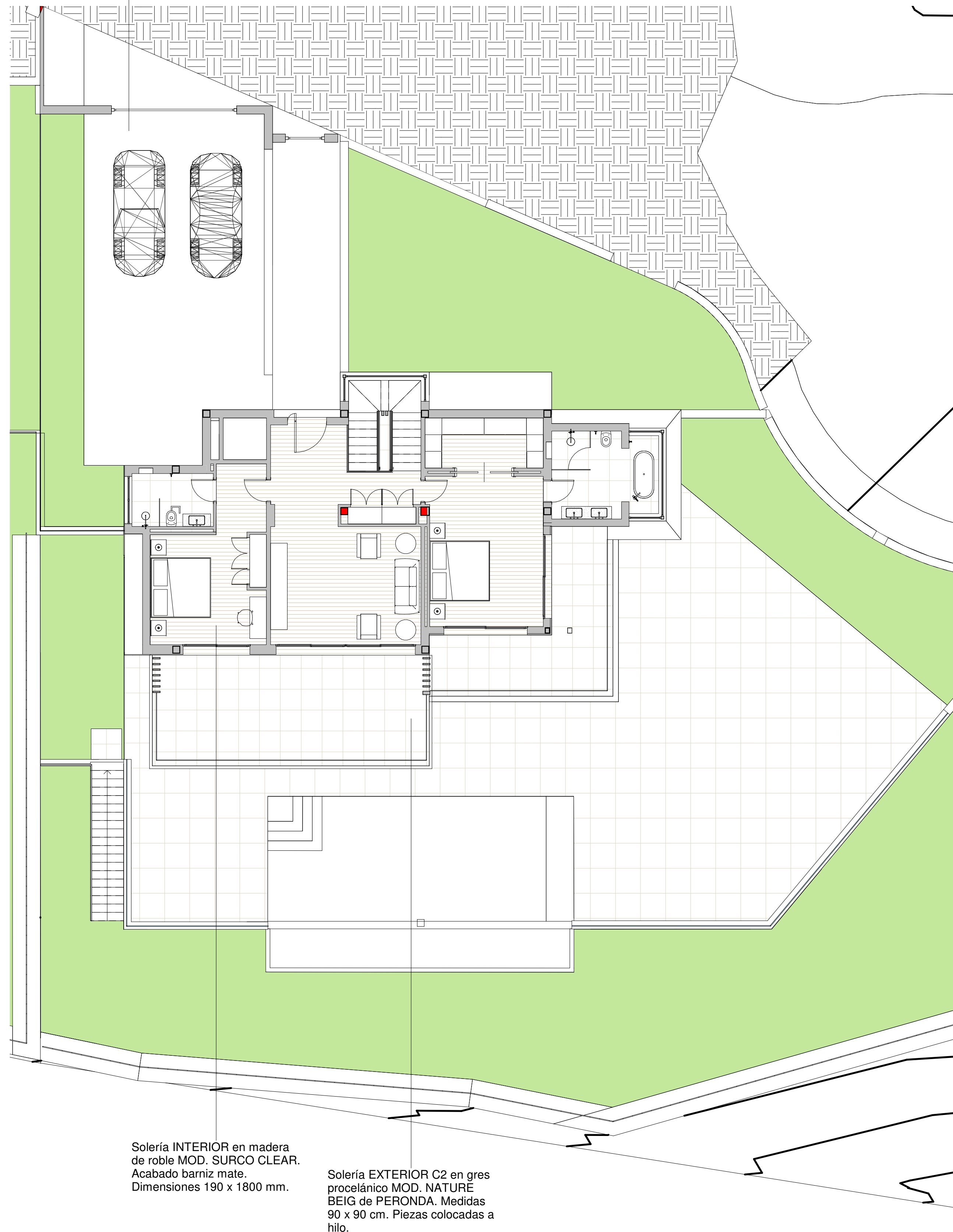
1 VC06 - Solados Planta alta 1:100
