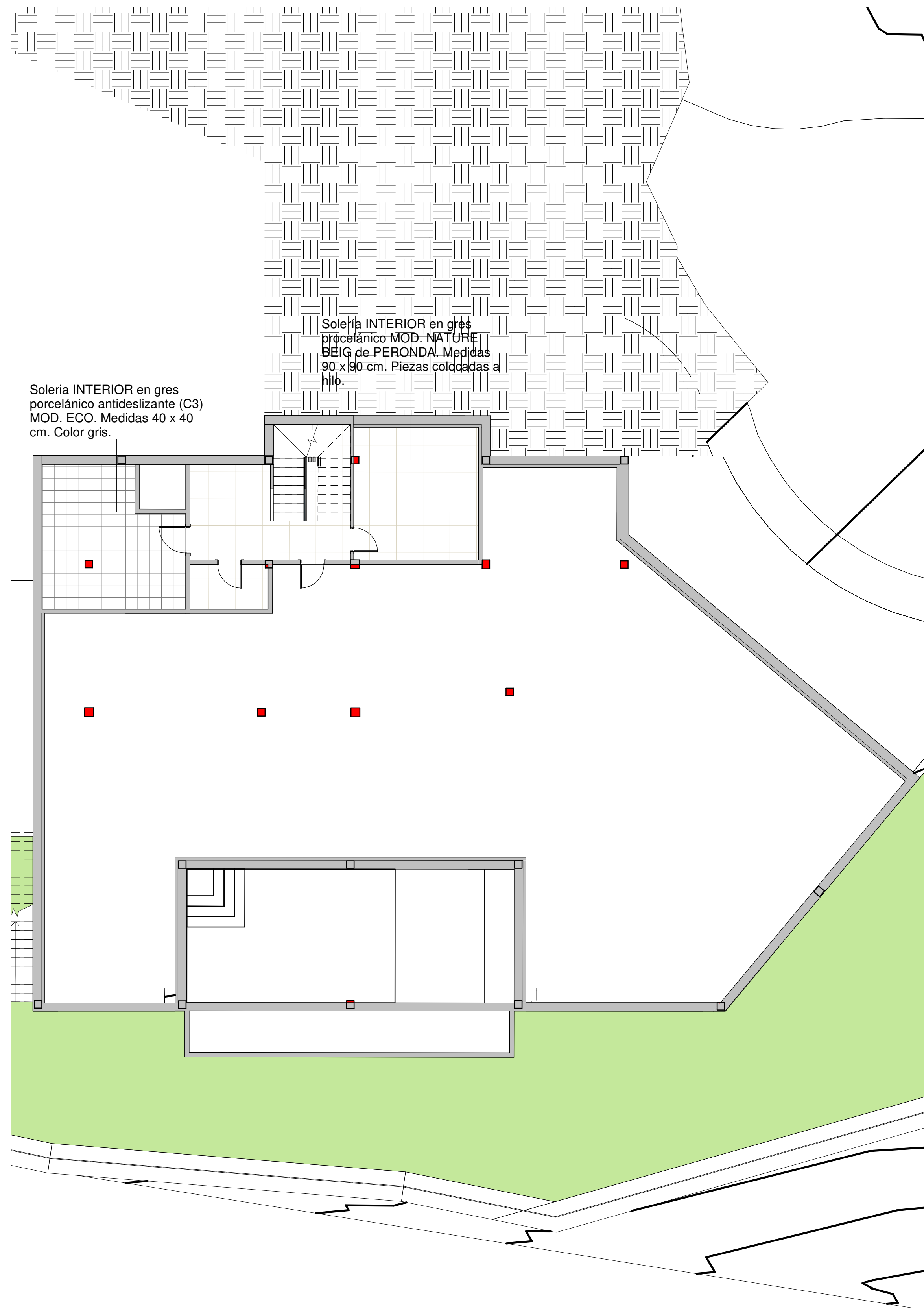
1 VC06 - Solados Planta sótano 1 : 100
